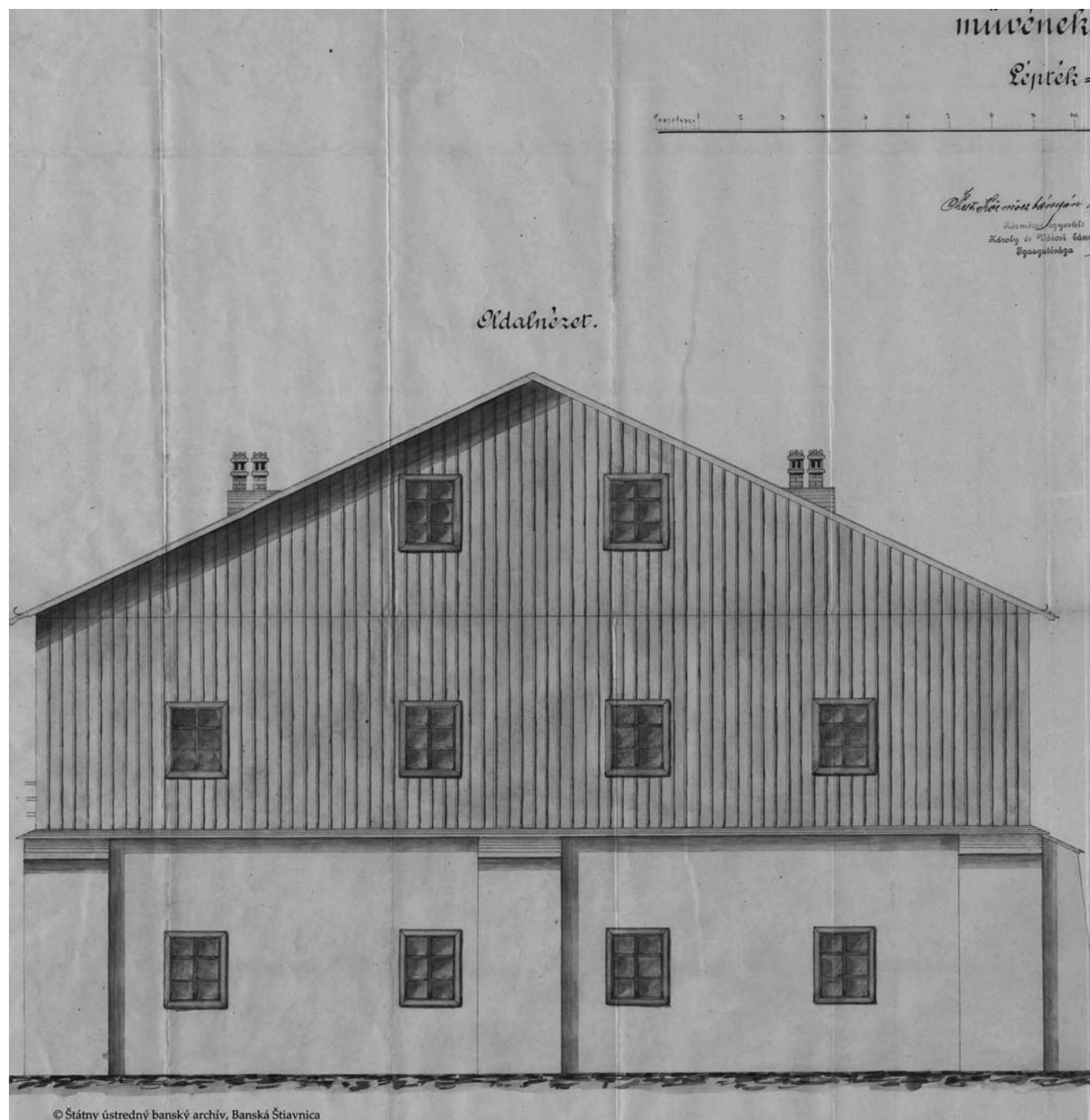
Budova úpravne rúd spojenej banskej spoločnosti Karol a mesta Kremnica, 1876 Slovenský banký archív v Banskej Štiavnici
