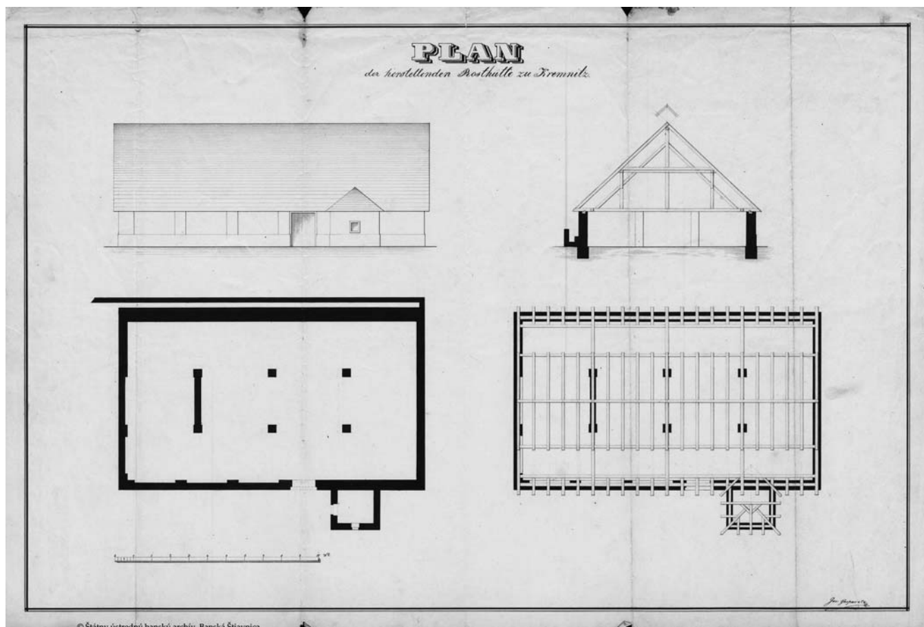
Plán na výstavbu budovy pražiarenskej huty v Kremnici, cca polovica 19. storočia Slovenský banký archív Banská Štiavnica
